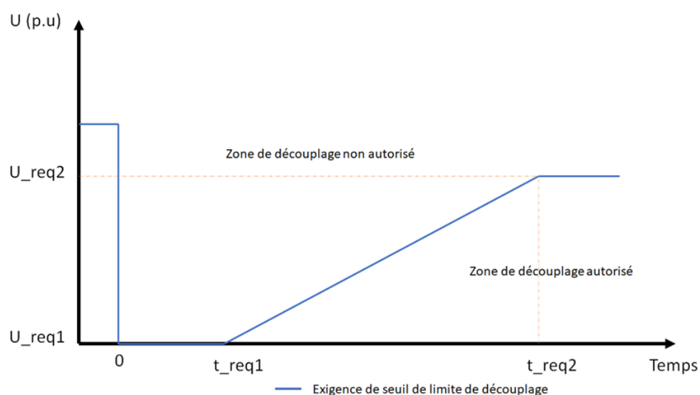
Figure 8 : Capacité de tenue aux creux de tension-Courbe temps/tension
