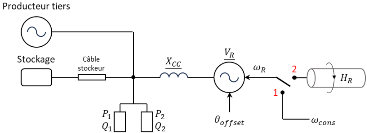
Figure 13 : modèle du réseau
