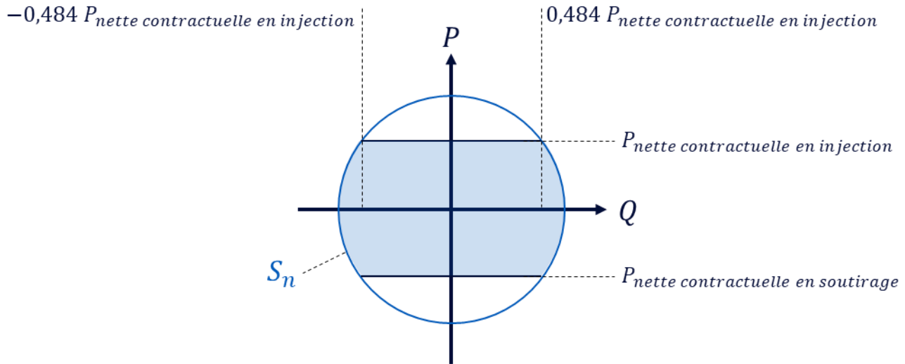
Figure 9 : Diagrammes PQ du stockage
