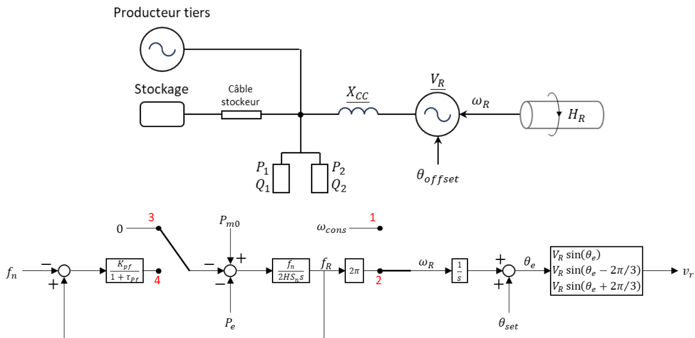
Figure 19 : modèle réseau pour la fiche 4
